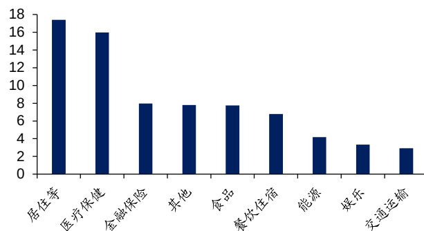
图3 美国 PCE 的主要分项权重对比 (%)
